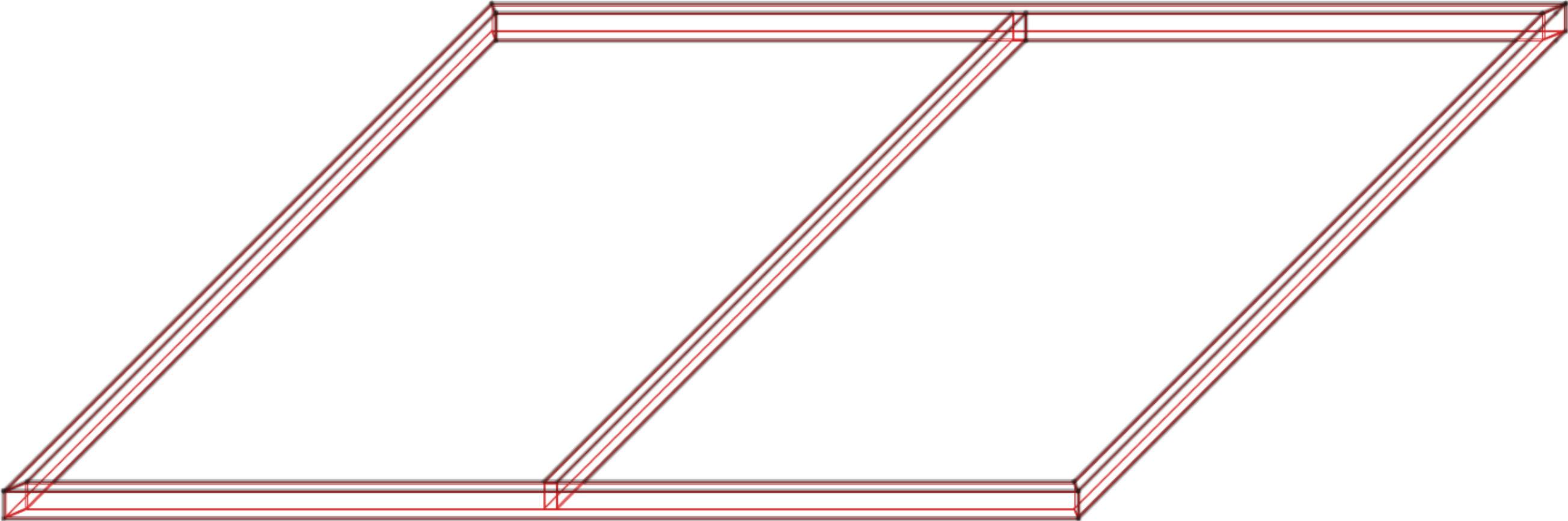
Рама 1565x1005 (вид DWG): линий/окружностей DWG 27, макс. отклонение от модели 0.003 мм
